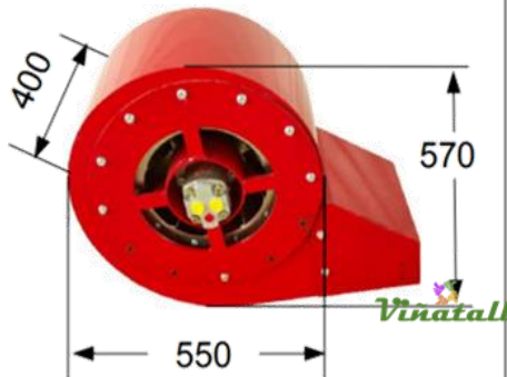
KIT TURBINE (hors ramasseuse)
